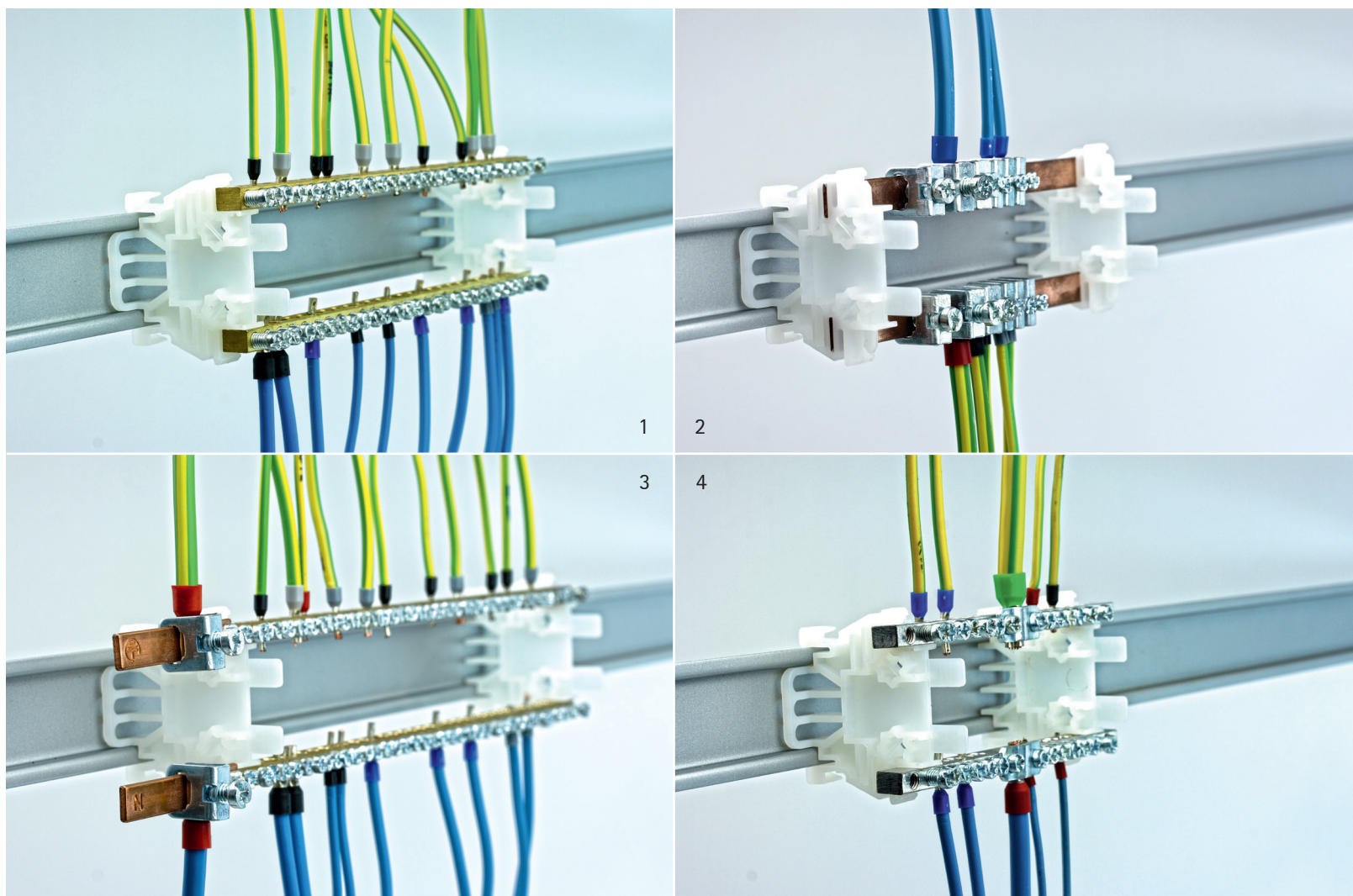
1 Aplikace s 870-XX mosaznou lištou | 2 Aplikace s plochou sběrnici a BKSG | 3 Aplikace s kombinací 870-XX lištou a plochou sběrnici 4 Aplikace s pozinkovanou svorkovou lištou
