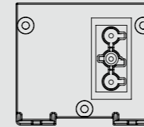
Endkappe mit Steckverbinder GST 18/3-Stecker, Strom Eingang
