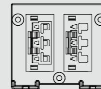
Endkappe mit 2x Steckverbinder Wago WINSTA /3-Buchse / Stecker Strom Ein / Ausgang
